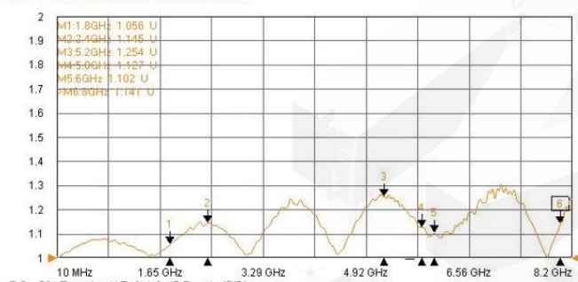
Tr1 S11 Refl SWR RefLvl: 1 U Res: 100 mV/Div
