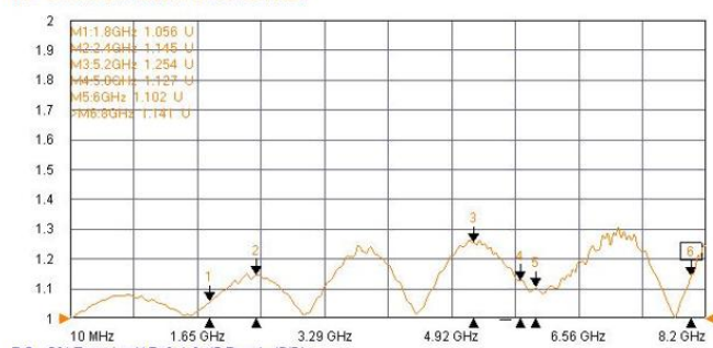
Tr1 S11 Refl SWR RefLvl: 1 U Res: 100 mU/Div
